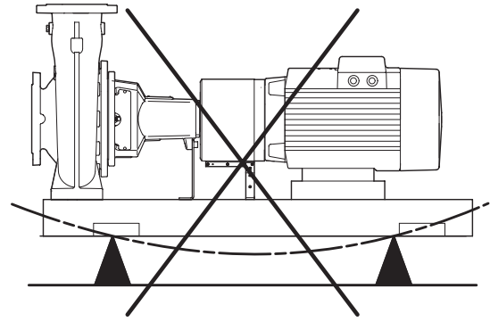
Рис. 8 Неправильный фундамент
