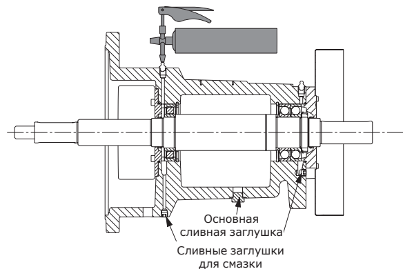
Рис. 28 Замена смазки
