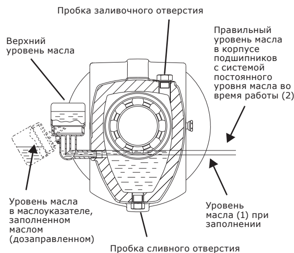
Рис. 18 Заливка масла
